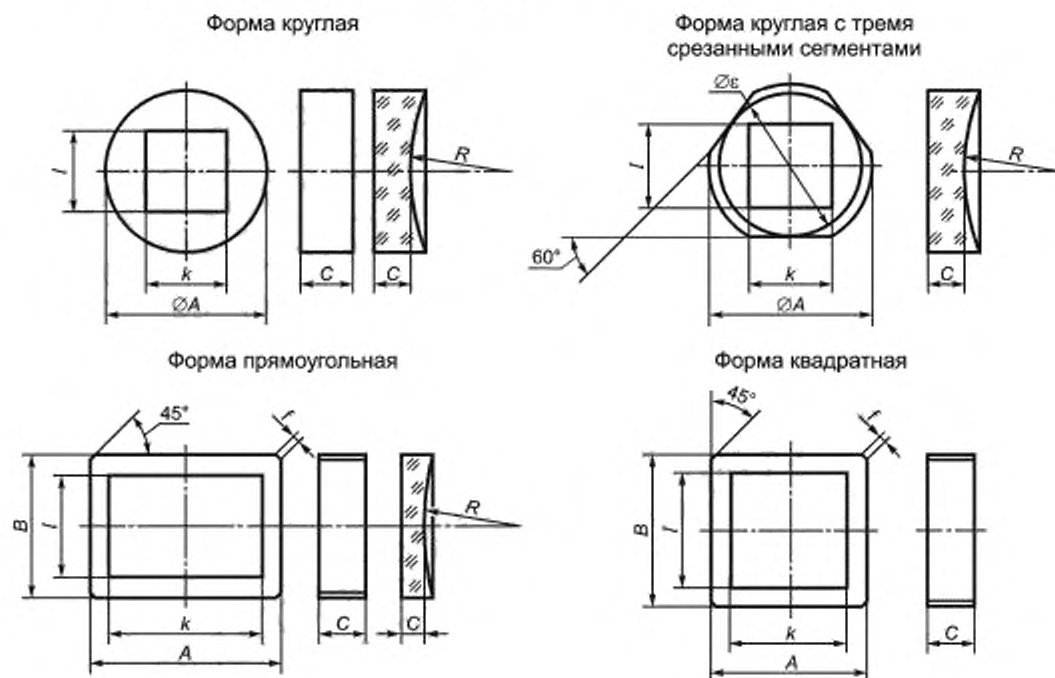
Рисунок 1 — Формы и размеры дифракционных решеток
