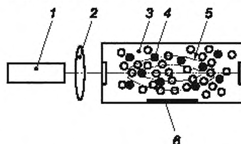
1 — перестраиваемый лазер; 2 — линза; 3 — ячейка; 4 — обнаруживаемый объект; 5 — ультразвук; 6 — микрофон
