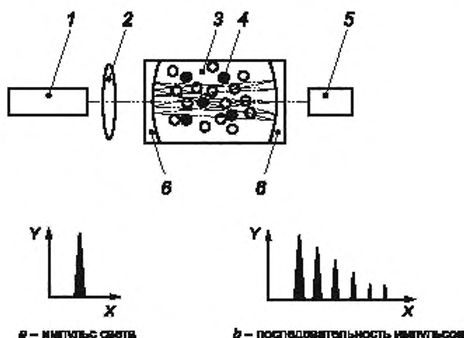
X — длина волны, Y — интенсивность, 1 — перестраиваемый лазер, 2 — линза; 3 — ячейка; 4 — обнаруживаемый элемент; 5 — фотодетектор, 6 — зеркало
