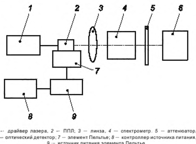
Рисунок 9 — Схема установки для измерения температурной зависимости длины волны генерации
