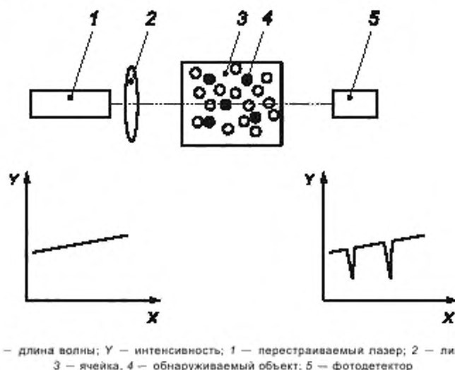
Рисунок 1 — Принцип работы измерительной TLAS-установки, применяемой для определения малой концентрации веществ методом лазерной абсорбционной спектроскопии (наблюдает два пика поглощения излучения)
