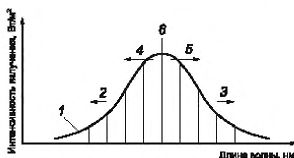
1 — огибающая усиления; 2 — изменение энергетического уровня из-за заполнения зоны; 3 — изменение запрещенной зоны из-за повышения температуры; 4 — изменение показателя преломления за счет эффекта носителя (плазмы); 5 — изменение показателя преломления при нагревании; 6 — моды резонатора
