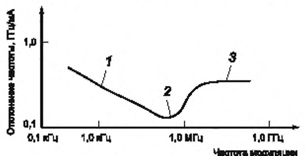
1 — нагрев (удлинение); 2 — провал; 3 — плазменный эффект (укорочение)
