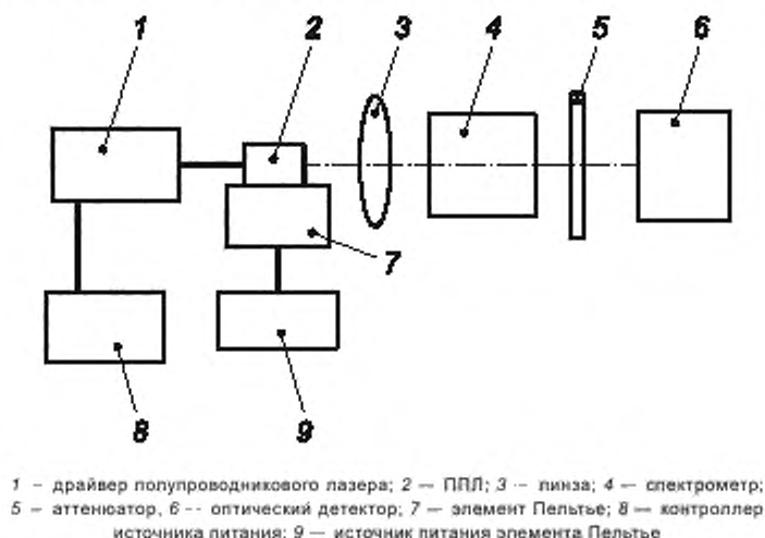
Рисунок 10 — Схема установки для измерения токовой зависимости длины волны генерации
