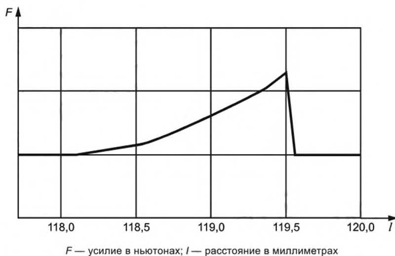
Рисунок С.3 — Пример графика зависимости усилия от перемещения
