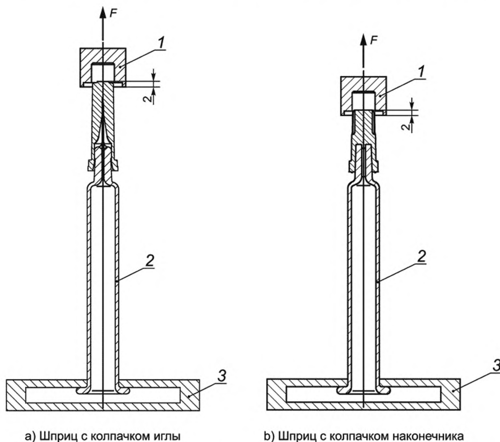
Рисунок G.6 — Примеры испытательного оборудования для определения усилия для снятия колпачка наконечника или защитного колпачка иглы (метод 1)
