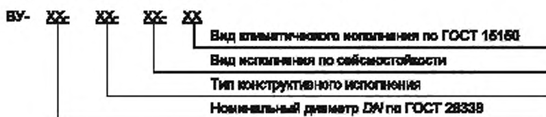
Рисунок 1 — Схема условного обозначения ВУ
