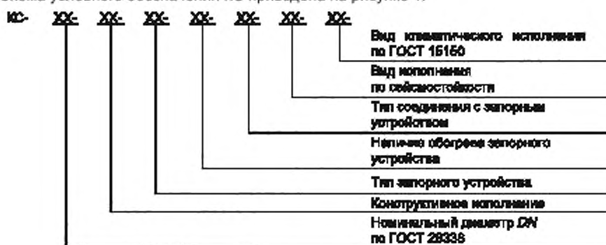
Рисунок 1 — Схема условного обозначения КС
