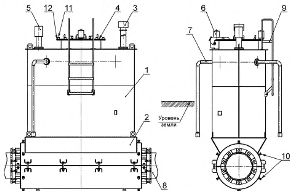
1 — отсек СИ; 2 — устройство фиксации; 3 — труба вытяжки воздуха; 4 — крышка; 5 — труба притока воздуха; 6 — запирающее устройство; 7 — труба кабельного ввода; 8 — трубопровод; 9 — лестница; 10 — устройство регулирования; 11 — поджимной болт; 12 — уплотнение
