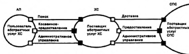
Рисунок 1 — Абстрактные услуги хранилища сообщений
