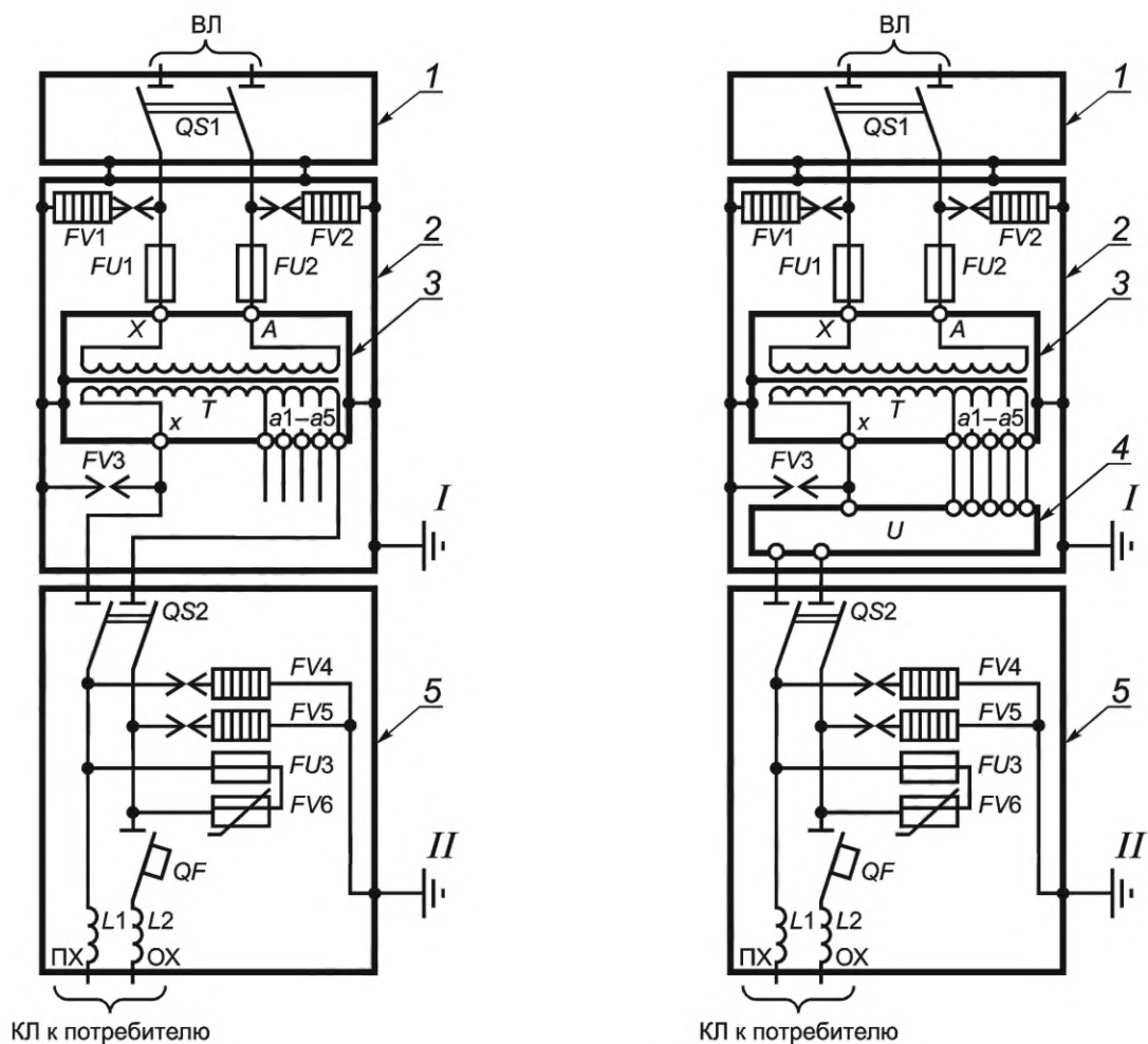
а) Без автоматического регулирования напряжения
