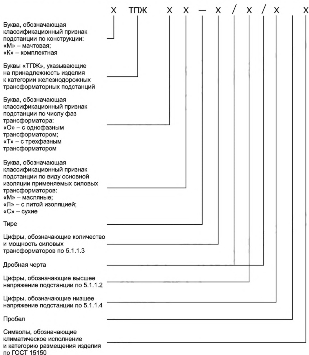
Рисунок 1 — Структурная схема условного обозначения подстанции
