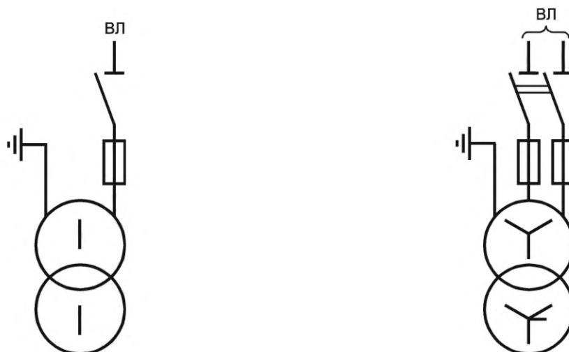
в) Схема для подстанций с высшим напряжением 27,5 кВ, воздушным вводом и однофазным трансформатором
