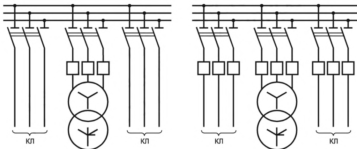
а) Схемы для подстанций с высшим напряжением 6, 10, 20 или 35 кВ со стационарным расположением выключателей
