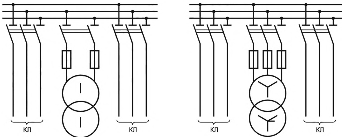
а) Схема для подстанций с высшим напряжением 6, 10, 20 или 35 кВ, воздушным или кабельным вводом и однофазным трансформатором
