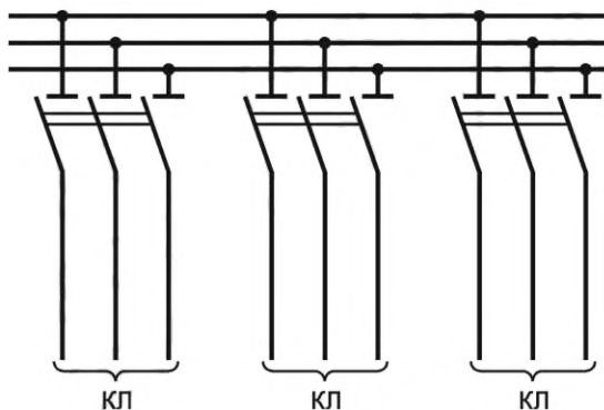
Рисунок 8 — Схема «секционирование разъединителями с ответвлением»
