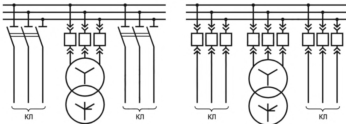
б) Схемы для подстанций с высшим напряжением 6, 10, 20 или 35 кВ с расположением выключателя на выкатном и (или) подъемно-опускном элементе
