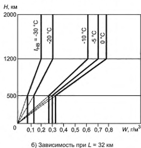
Рисунок Е.2 — Зависимость водности от вертикальной протяженности зоны обледенения
