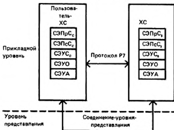
Рисунок 2 — Модель протокола доступа ХС
