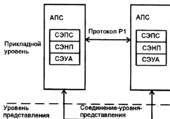
Рисунок 5 — Модель протокола передачи СПС
