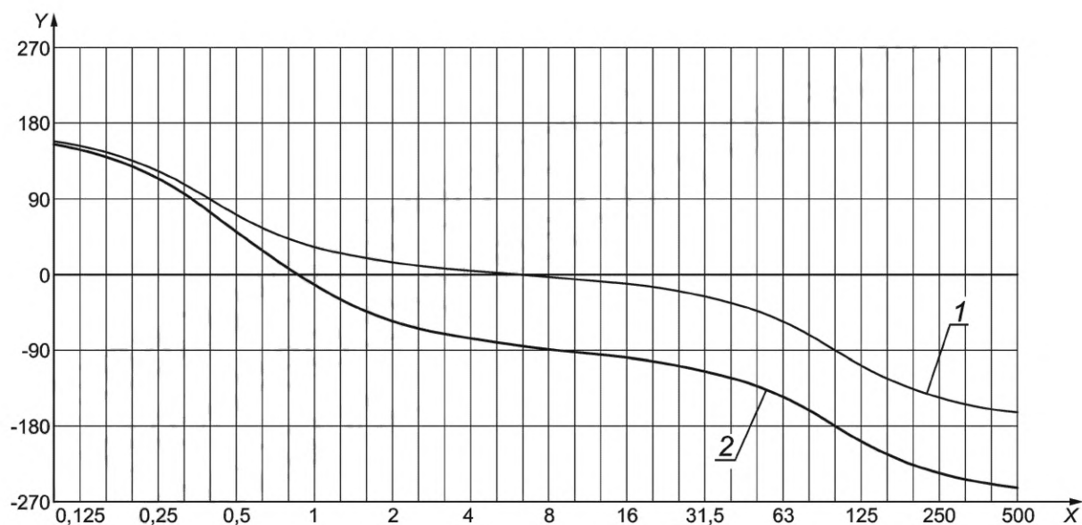
Рисунок В.8 — Фаза функции частотной коррекции W_e по ГОСТ 31191.1
