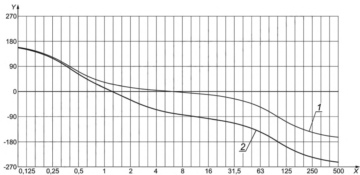
Рисунок В.6 — Фаза функции частотной коррекции W_d по ГОСТ 31191.1
