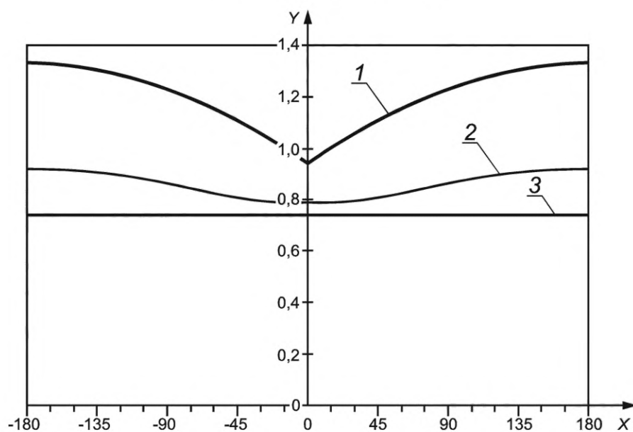
X — фазовый сдвиг гармоники, град; Y — фазовый сдвиг гармоники; 1 — пиковое значение, \text{м/с}^2 ; 2 — доза вибрации, \text{м/с}^{1.75} ; 3 — среднеквадратичное значение, \text{м/с}^2
