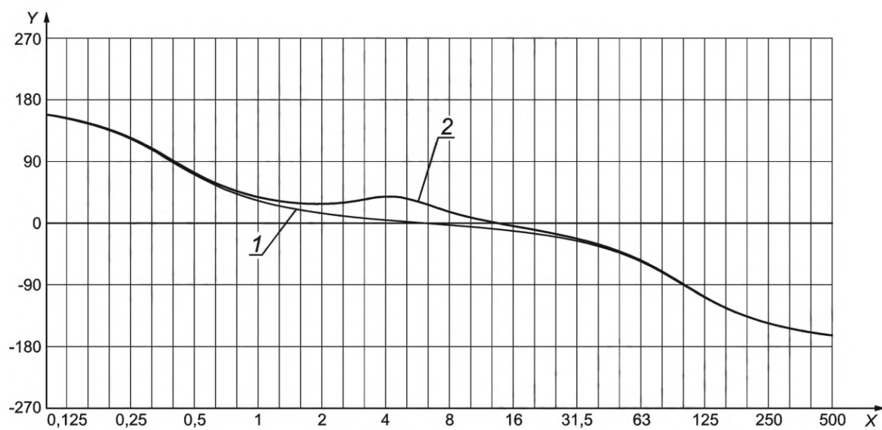
Рисунок В.14 — Фаза функции частотной коррекции W_j по ГОСТ 31191.1
