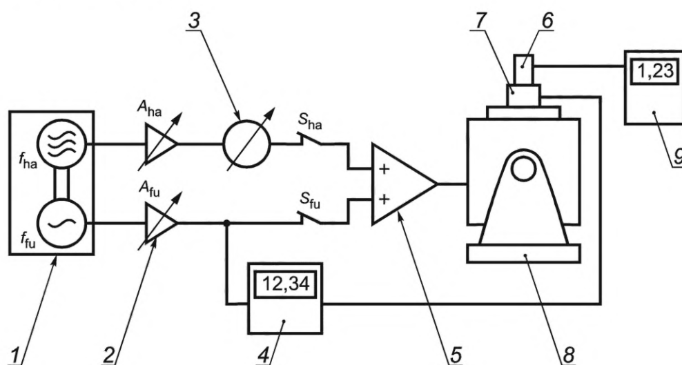
1 — двухканальный генератор сигналов с контролируемым сдвигом фаз; 2 — усилитель с регулируемым коэффициентом усиления; 3 — фазовращатель; 4 — фазометр; 5 — сумматор с усилителем мощности; 6 — преобразователь вибрации; 7 — эталонный акселерометр; 8 — вибростенд; 9 — виброметр
