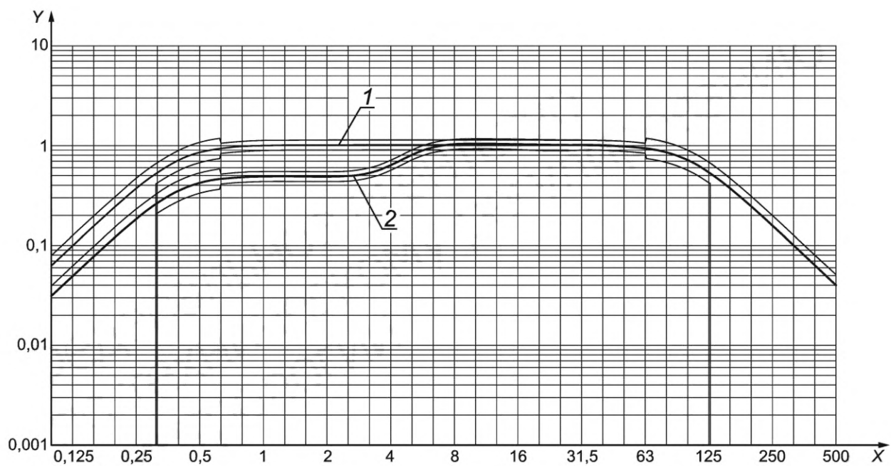
Рисунок В.13 — Модуль функции частотной коррекции W_j по ГОСТ 31191.1
