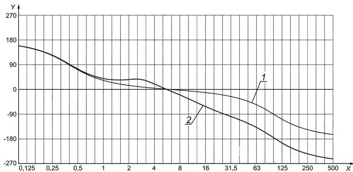
Рисунок В.16 — Фаза функции частотной коррекции W_k по ГОСТ 31191.1
