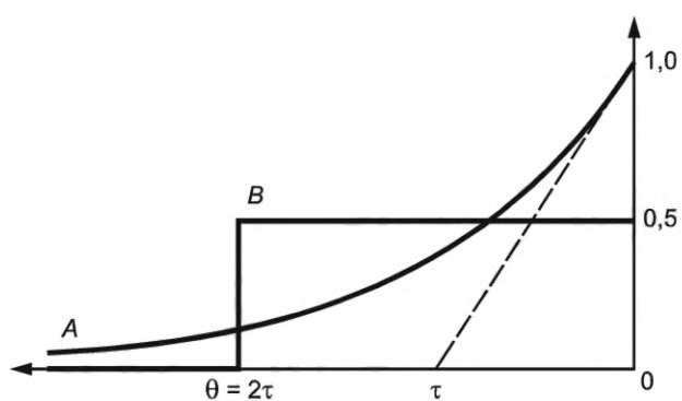
Рисунок D.3 — Временные весовые функции, обеспечивающие приблизительную эквивалентность результатов измерений максимального кратковременного среднеквадратичного значения скорректированного ускорения для импульсных сигналов
