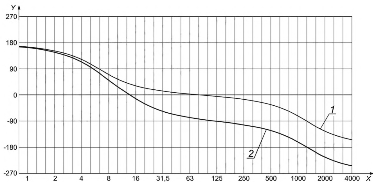
Рисунок В.12 — Фаза функции частотной коррекции W_h по ГОСТ 31192.1
