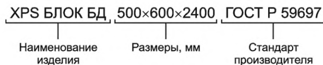
Рисунок 1 — Пример условного обозначения XPS-блоков
