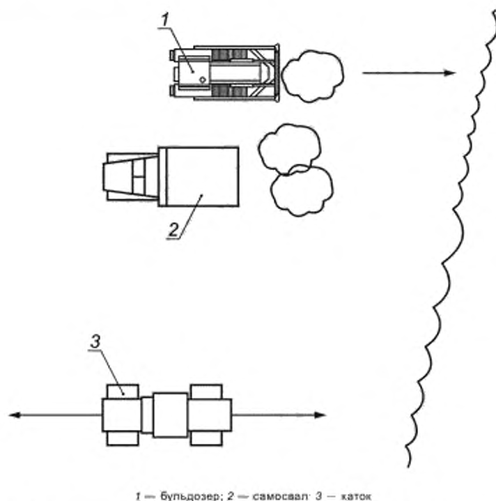
Рисунок А.1 — Принципиальная схема проведения работ при отсыпке песка в основании насыпи (выгрузка песка, разравнивание, уплотнение)
