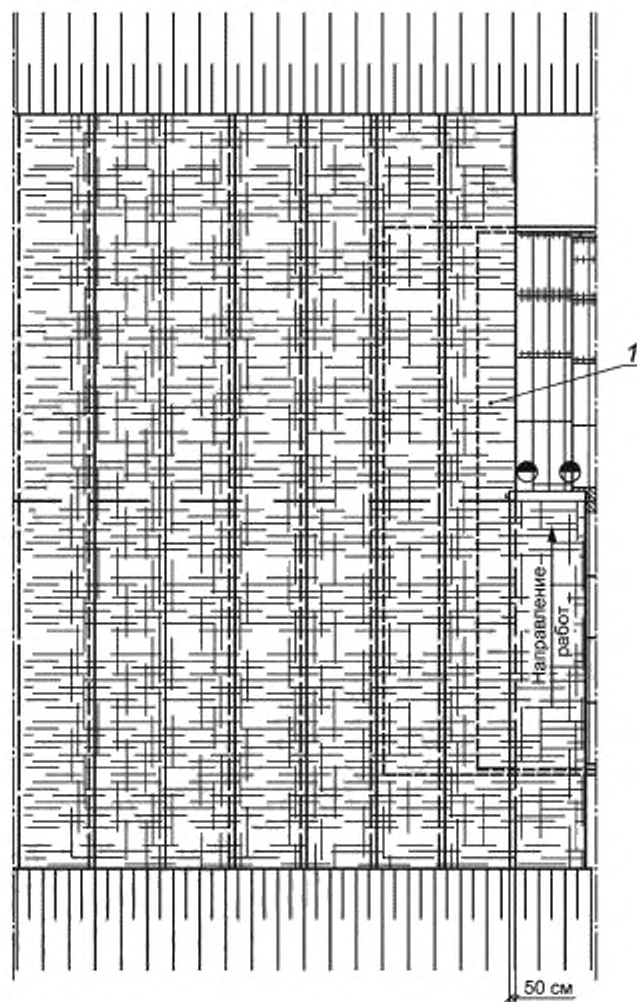
1 — геосинтетический материал
