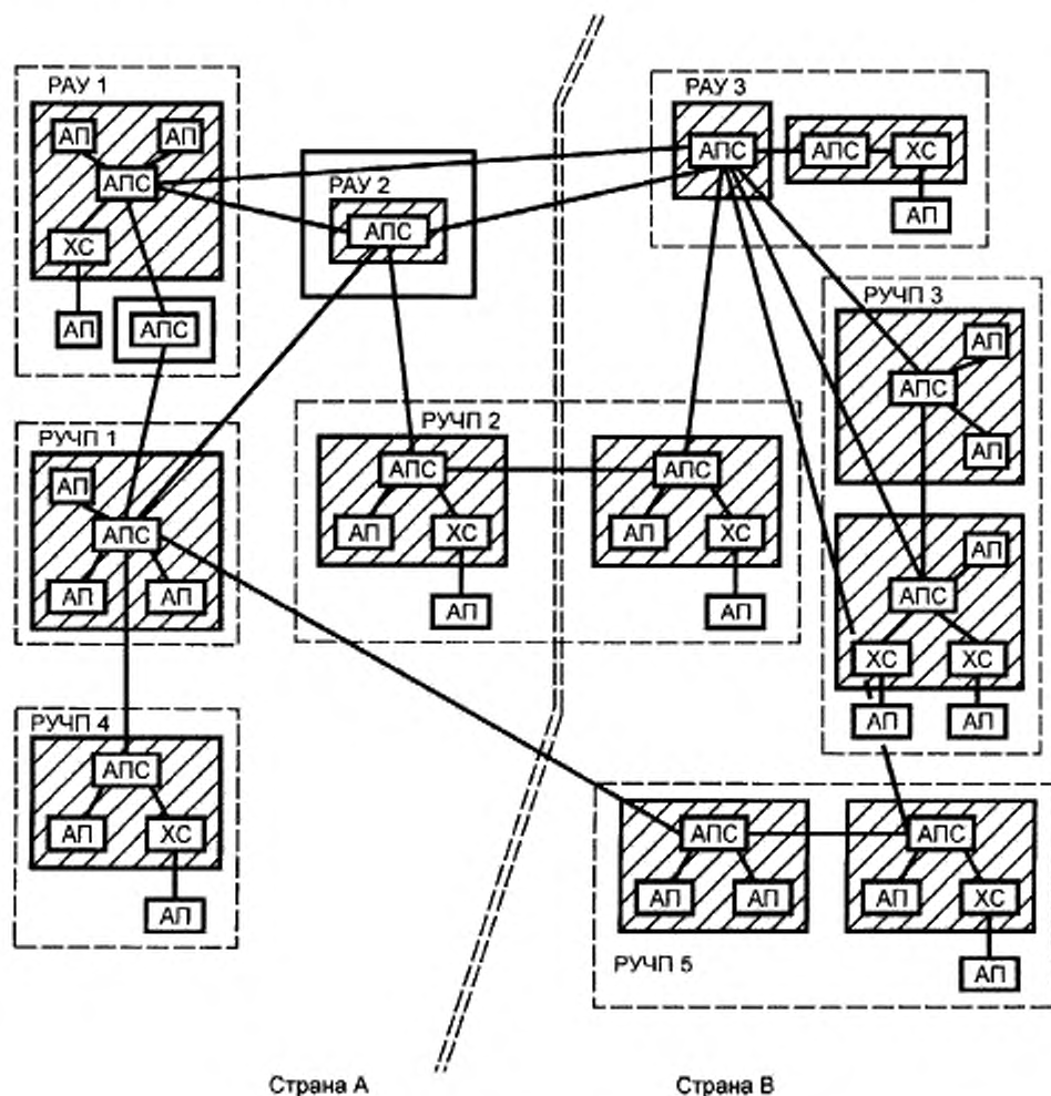
Рисунок 5 — Взаимосвязи между регионами управления
