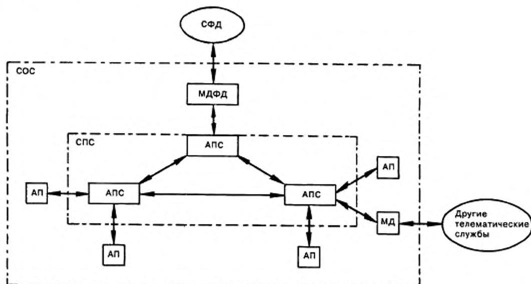
Рисунок 10 — Функциональная модель взаимодействия СОС-СФД
