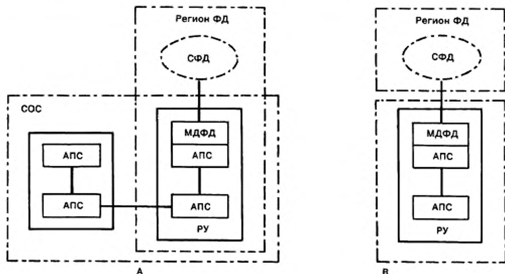
Рисунок 11 — Конфигурации взаимосвязи служб ОС/ФД
