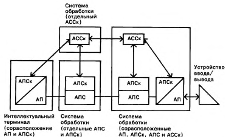
Рисунок 13 — Физические конфигурации взаимодействия справочников СОС
