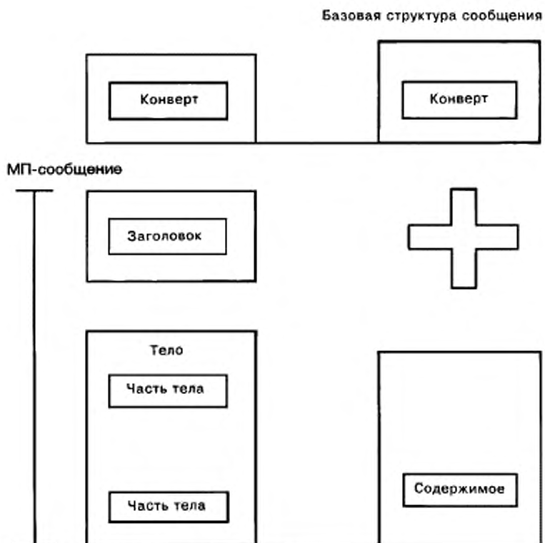
Рисунок 8 — Структура МП-сообщения
