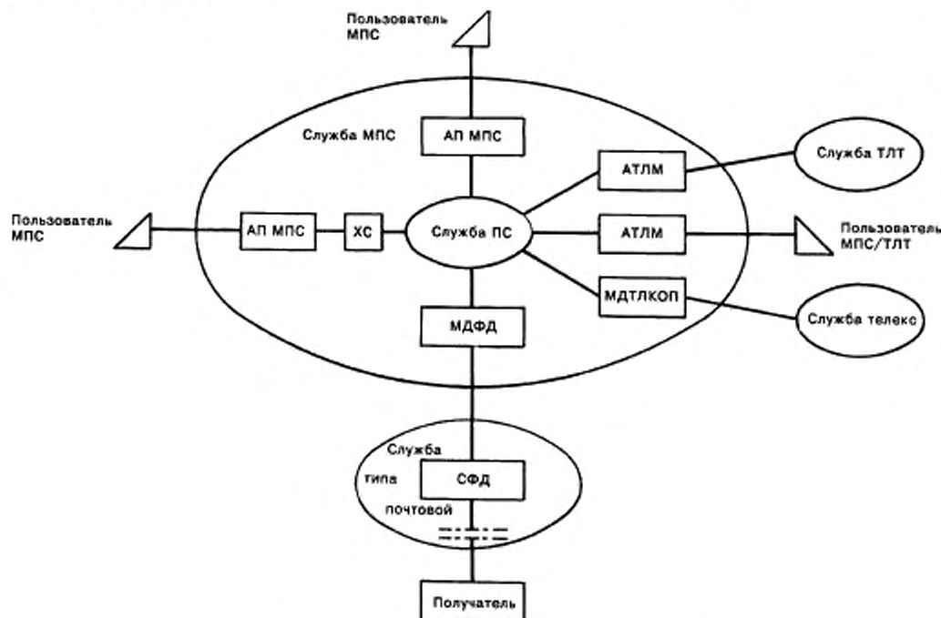
Рисунок 7 — Функциональная модель службы МПС
