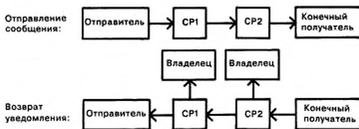
Рисунок 15 — Уведомления СР
