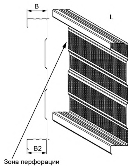
Рисунок А.4 — Рядовой акустический сэндвич-профиль
