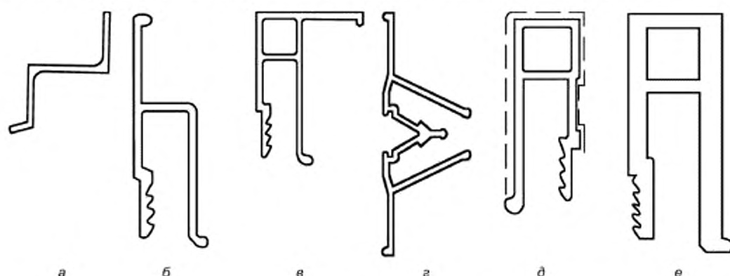
а — Z-образный алюминиевый профиль (отбойник); б — H-образный алюминиевый облегченный профиль; в — универсальный алюминиевый профиль; г — соединительный алюминиевый профиль; д — П-образный алюминиевый профиль; е — стеновой ПВХ профиль
