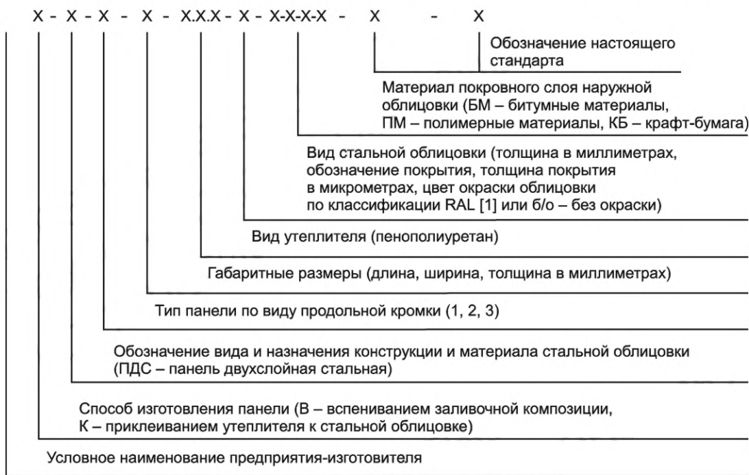
Рисунок 3 — Схема обозначения панелей
