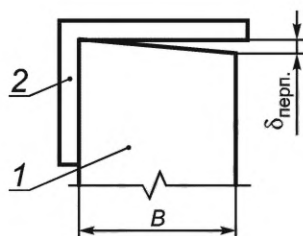
Рисунок 6 — Схема определения неперпендикулярности сторон
