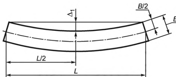
Рисунок 5 — Схема определения непрямолинейности продольных кромок панели
