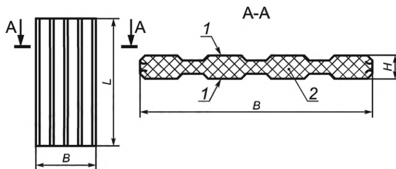
Рисунок 2 — Трехслойная панель
