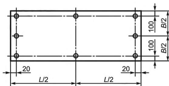
Рисунок 4 — Расположение точек измерения толщины панели
