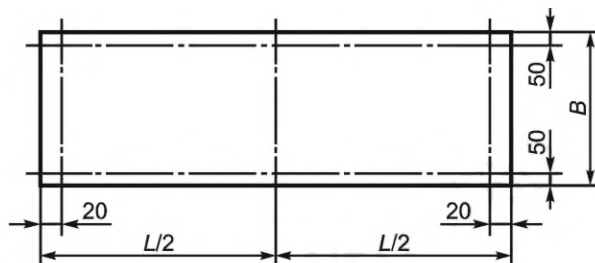
Рисунок 3 — Расположение мест измерения длины и ширины панели
