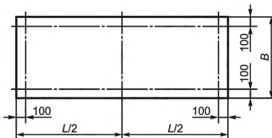
Рисунок 7 — Расположение мест проверки неплоскостности панели
