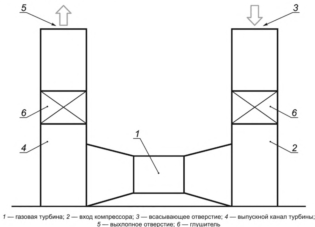
Рисунок В.1 — Определение основных источников шума, газовая турбина
