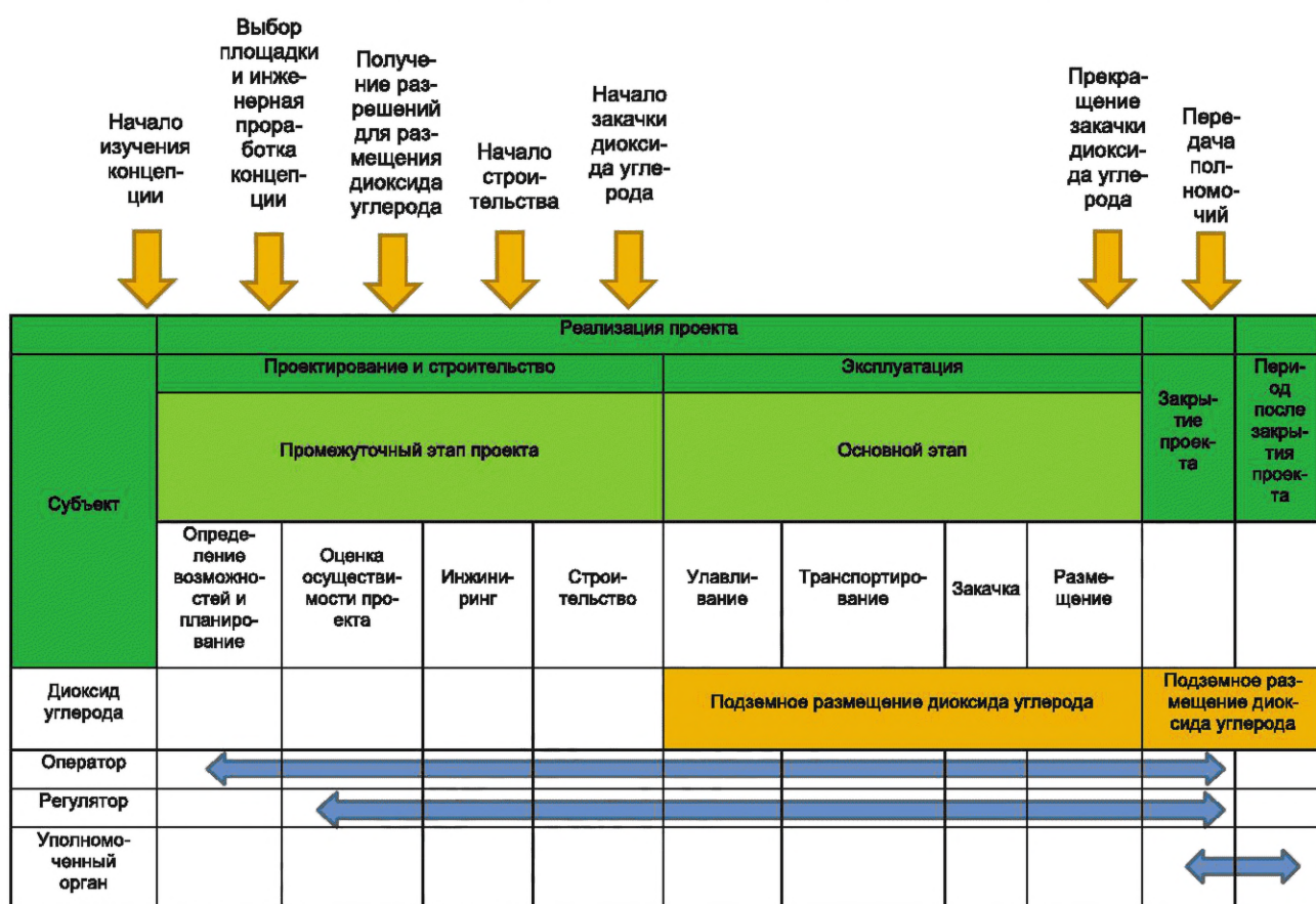
Рисунок В.1 — Жизненный цикл проекта по улавливанию и размещению диоксида углерода
