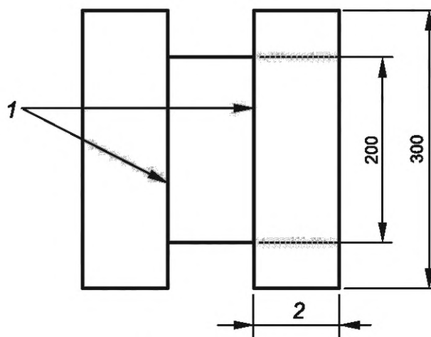
Рисунок 2 — Нарезка образцов
