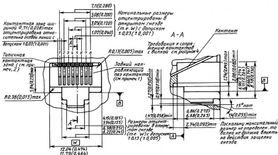
Рисунок 5 — Механические характеристики гнезда
