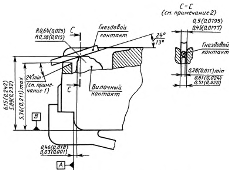
Рисунок 4 — Спецификация контактов гнезда и вилки
