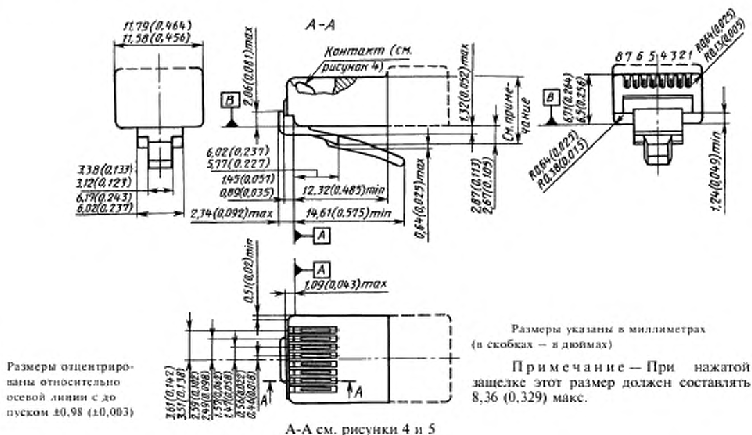
Рисунок 3 — Механические характеристики вилки
