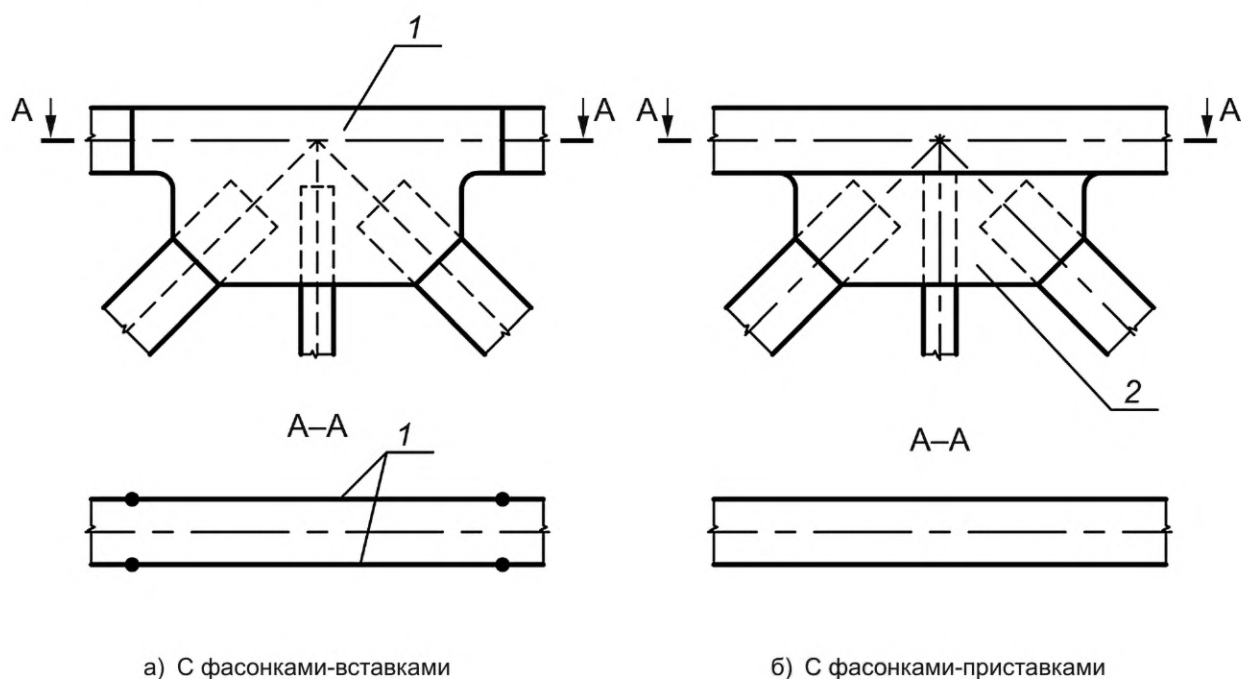
Рисунок 11.1 — Типы узлов главной фермы
