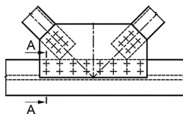
Рисунок В.3 — Расположение проверяемого на выносливость расчетного сечения А—А по основному металлу в сечении брутто по первому ряду высокопрочных болтов в прикреплении фасонки к нестыкуемым в данном узле поясам сплошных балок и элементам решетчатых форм
