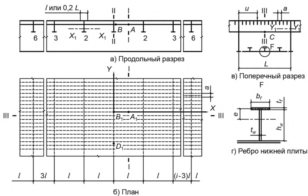
Рисунок Г.1 — Коробчатое пролетное строение
