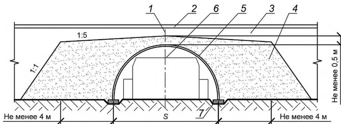
Рисунок 3 — Конструкция грунтовой обоймы замкнутого сооружения
