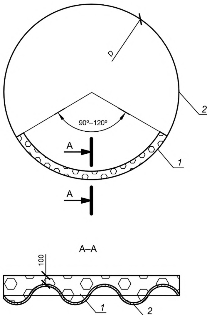
Рисунок 5 — Расположение лотка в конструкции из МГЭ
