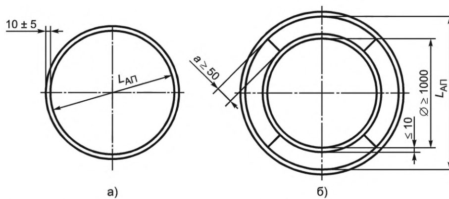
Рисунок 7 — Антифрикционные пластины для сферических поверхностей скольжения
