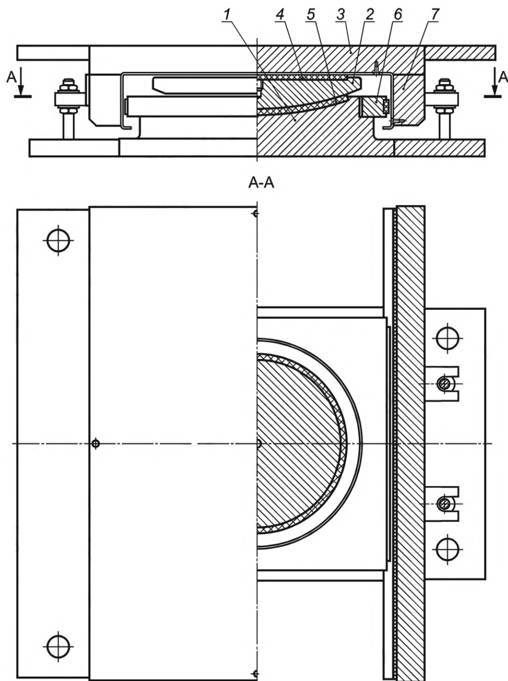
1 — постель балансира; 2 — балансир (шаровый сегмент); 3 — скользящая плита; 4, 5 — антифрикционная пластина; 6 — кольцо; 7 — направляющая
