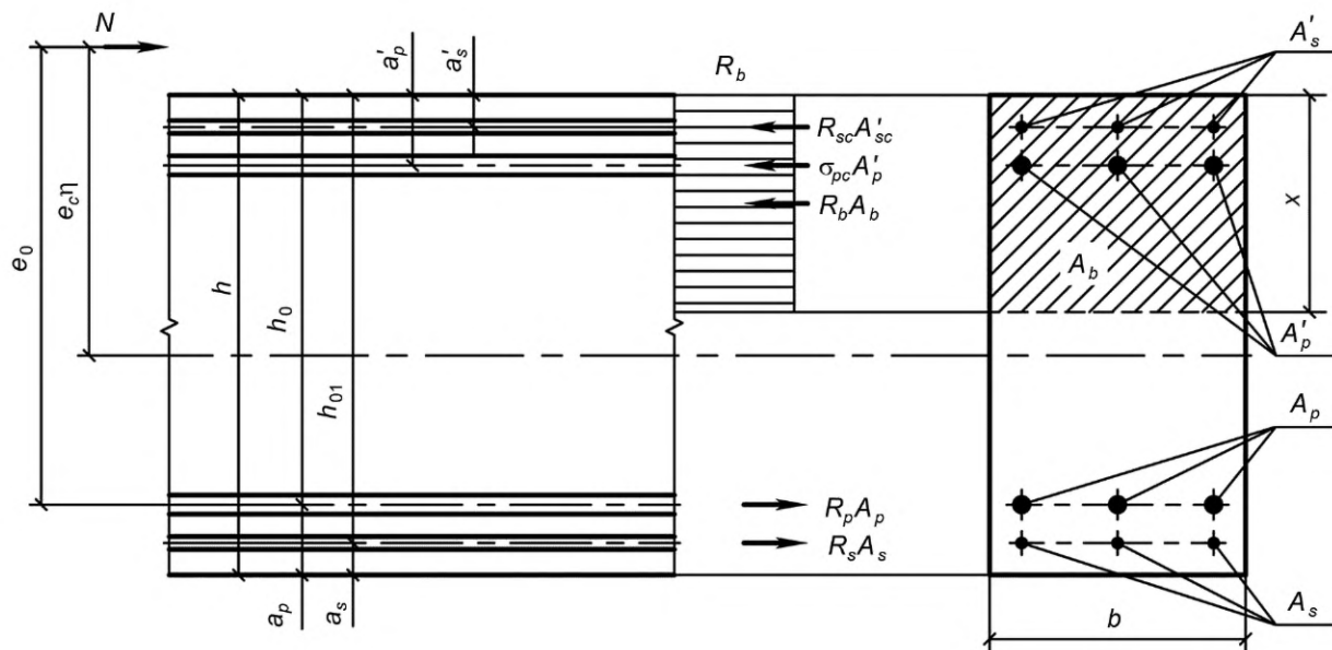
Рисунок 7.3 — Схема усилий и эпюра напряжений в сечении, нормальном к продольной оси внецентренно сжатого железобетонного элемента, при расчете его по прочности
