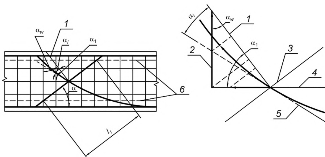
1 — нормаль; 2 — хомут; 3 — наклонное сечение; 4 — продольная арматура; 5 — касательная к пучку; 6 — вут
