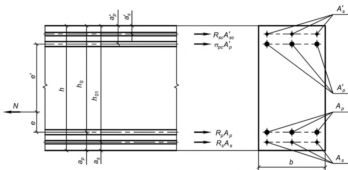
а) Продольная сила N приложена между равнодействующими усилий в арматуре
