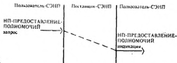
Рисунок 6 — Примитивы услуги НП-ПРЕДОСТАВЛЕНИЕ-ПОЛНОМОЧИИ
