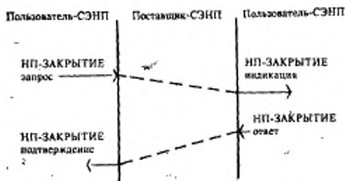
Рисунок 3 — Примитивы услуги НП-ЗАКРЫТИЕ
