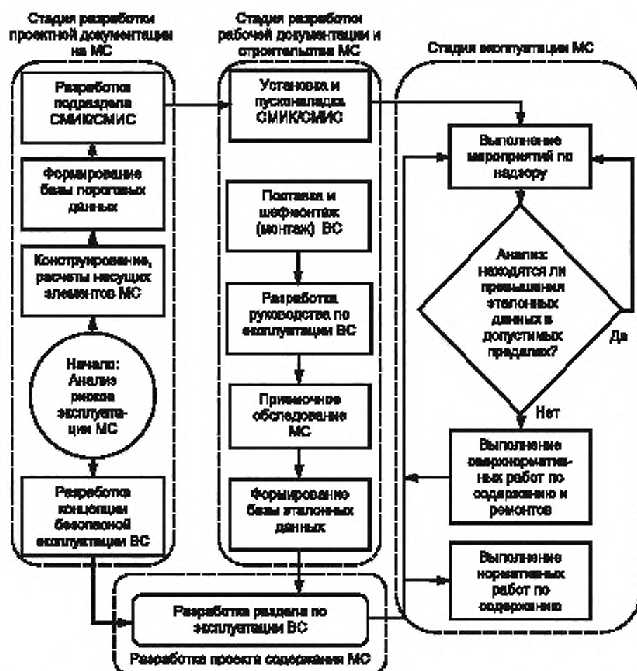
Рисунок 1 — Организационная структура мероприятий по подготовке и проведению эксплуатации ВС автодорожных мостов
