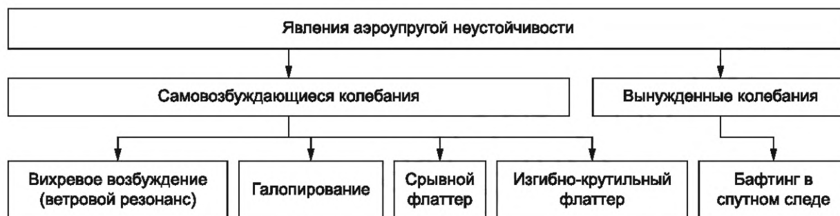
Рисунок 1 — Явления аэроупругой неустойчивости
