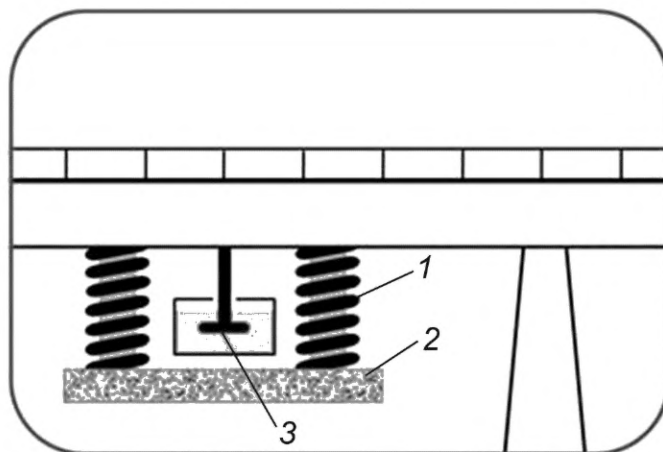
Рисунок Г.3 — Динамический гаситель колебаний (TMD — демпфер)
