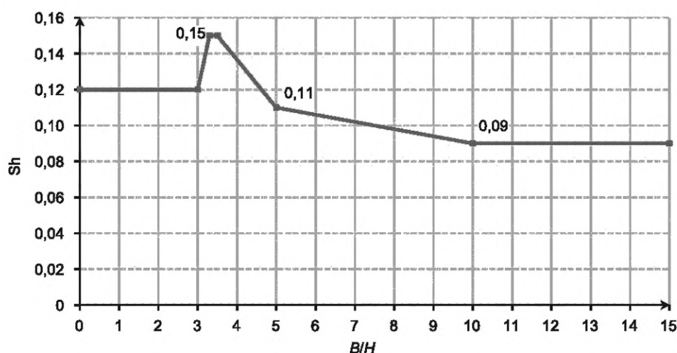
Рисунок 3 — Зависимость числа Струхала от B/H
