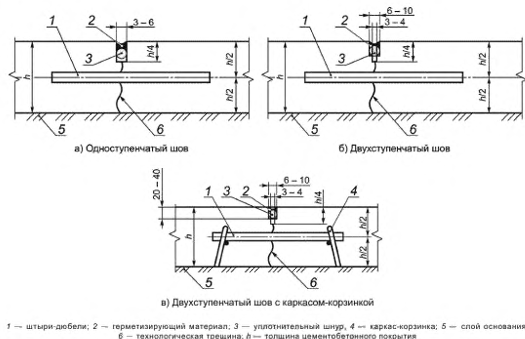
Рисунок 5 — Конструкции поперечных швов сжатия
