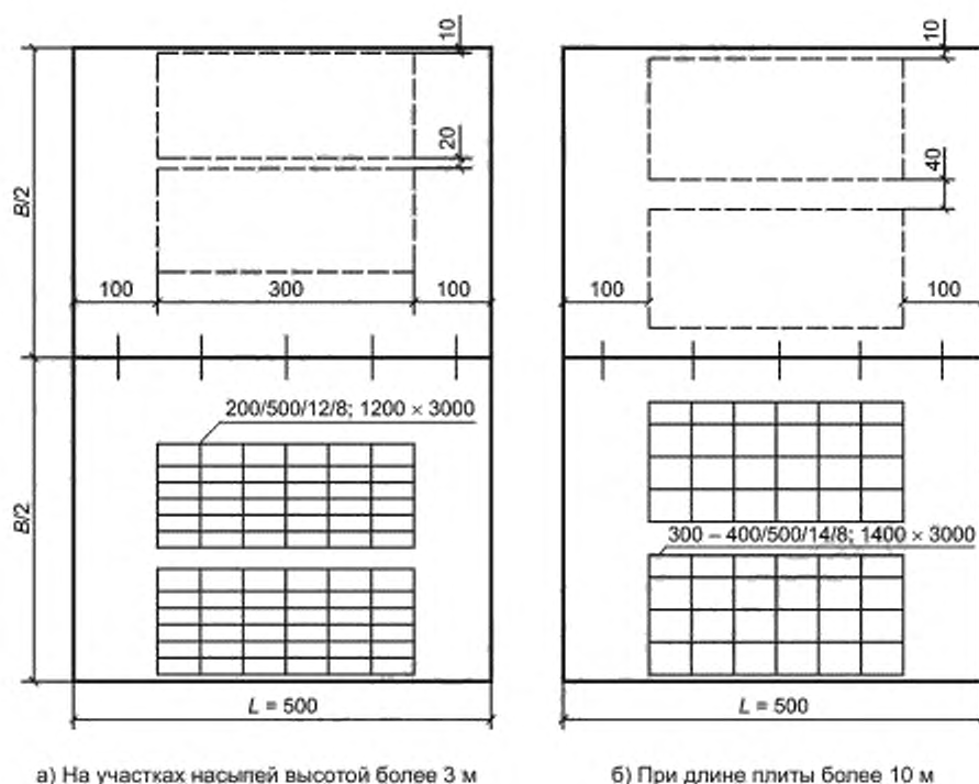
Рисунок 9 — Схемы армирования цементобетонных плит
