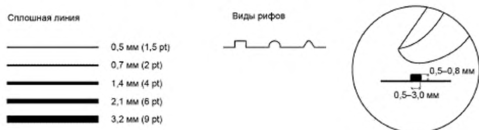
Рисунок 17 — Сплошная линия
