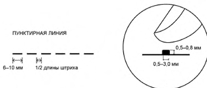
Рисунок 18 — Пунктирная линия
