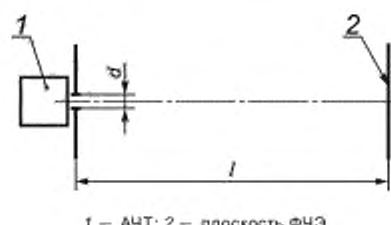
Рисунок Д.1 — Схема формирования потока излучения, создаваемого высокотемпературным АЧТ
