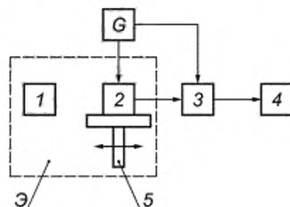
1 — источник излучения; 2 — испытуемый образец; 3 — БЭО; 4 — ПК; 5 — система перемещения; G — источник питания; Э — светозащитный экран
