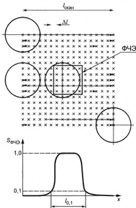
Рисунок 10 — Схема сканирования ФЧЗ ФПУ
