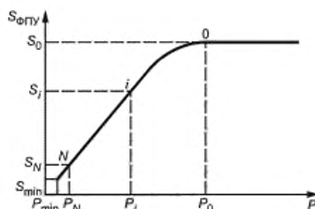
Рисунок 6 — График зависимости сигнала с ФЧЗ (среднего значения сигнала ФЧЗ ФПУ или зоны ФПУ по недефектным ФЧЗ) от потока излучения (или плотности потока)
