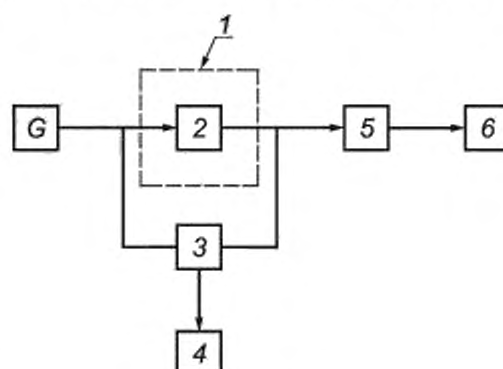
1 — испытуемый образец; 2 — МКС; 3 — измерительная оснастка; 4 — мультиметр; 5 — измерительная оснастка; 6 — мультиметр; G — источник питания
