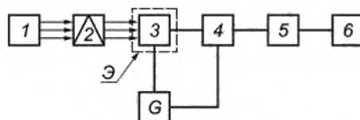
1 — источник излучения; 2 — модулятор (при необходимости); 3 — испытуемый образец; 4 — БЗО; 5 — ПК; 6 — специализированное ПО; G — источник питания; Э — светозащитный экран (при необходимости)
