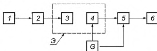
1 — светодиод; 2 — аттенуатор; 3 — конденсор (при необходимости); 4 — испытуемый образец; 5 — БЗО; 6 — ПК; G — источник питания; Э — светозащитный экран
