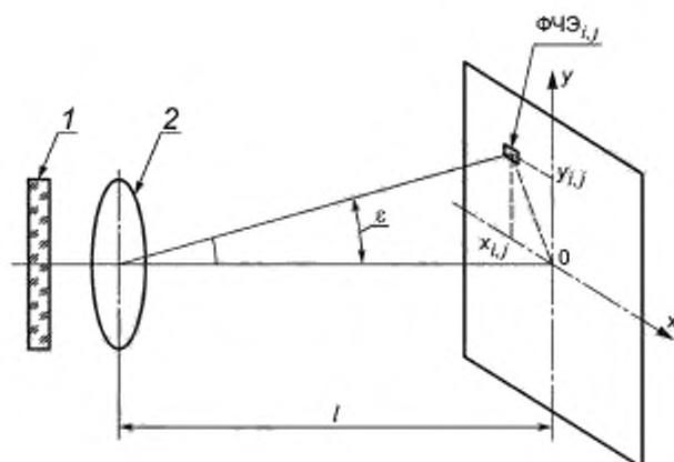
1 — входное окно, 2 — отверстие холодной диафрагмы
