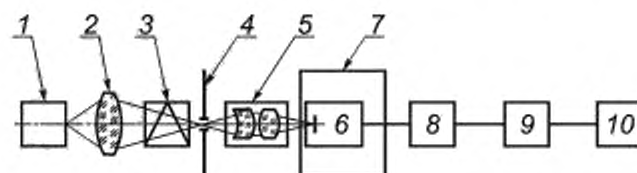
1 — источник излучения; 2 — конденсор; 3 — заслонка/модулятор; 4 — диафрагма; 5 — оптический зонд; 6 — испытуемый образец; 7 — координатный столик; 8 — БЗО; 9 — ПК; 10 — специализированное ПО
