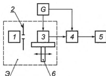
1 — источник излучения; 2 — набор сменных диафрагм; 3 — испытуемый образец; 4 — БЗО; 5 — ПК; 6 — система перемещения; G — источник питания; Э — светозащитный экран
