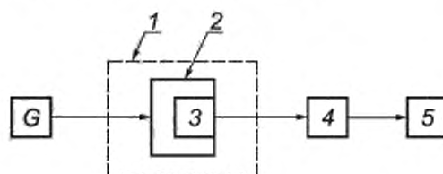
1 — испытываемый ФПУ; 2 — МКС; 3 — термодатчик; 4 — измерительная оснастка; 5 — вольтметр или другой регистрирующий прибор (система); G — источник питания МКС
