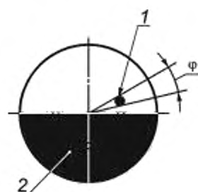
1 — диафрагма АЧТ; 2 — модулятор
