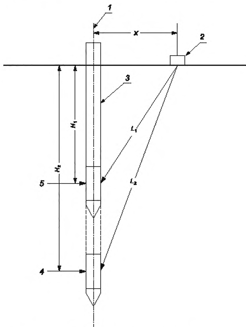
1 — ось зонда; 2 — ударная балка; 3 — штанга зонда; 4 — зонд на глубине H_2 ; 5 — зонд на глубине H_1
