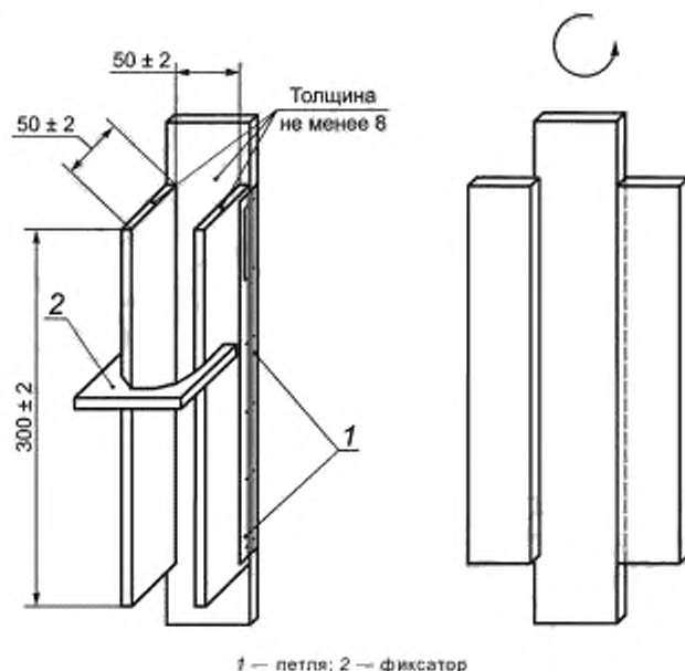
Рисунок А.1 — Форма из древесно-слоистой плиты
