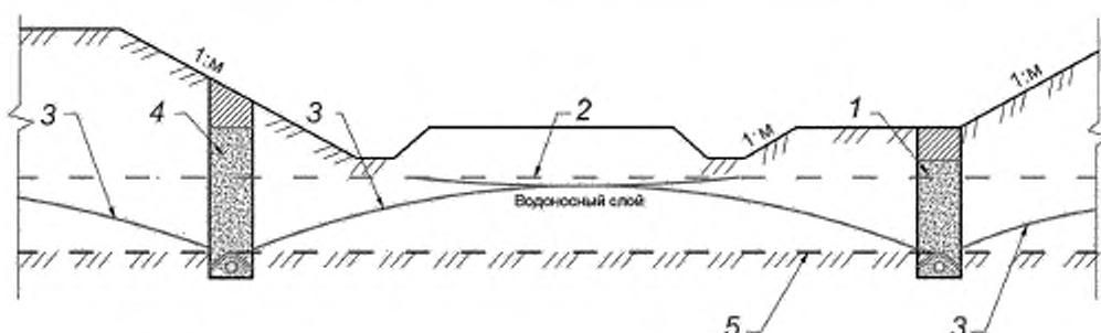
1 — заливный дренаж, устроенный на полке; 2 — уровень грунтовых вод до понижения; 3 — кривая депрессии после устройства дренажа; 4 — заливный дренаж, устроенный на откосе выемки; 5 — водоупорный слой
