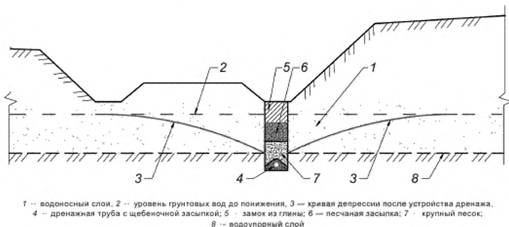
Рисунок 11 — Односторонний подкюветный дренаж глубокого заложения совершенного типа
