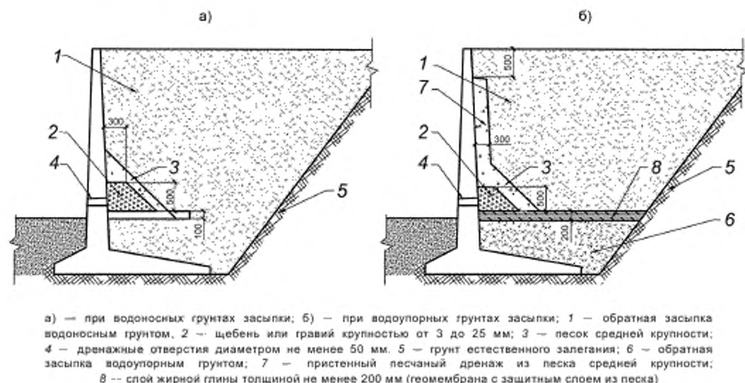
Рисунок 14 — Схемы застенных дренажей
