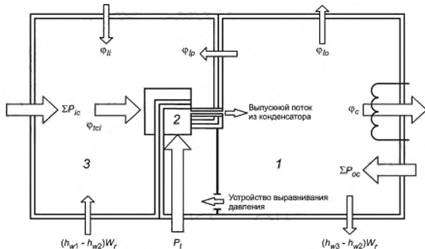
1 — внешнее отделение; 2 — испытуемое оборудование; 3 — внутреннее отделение
