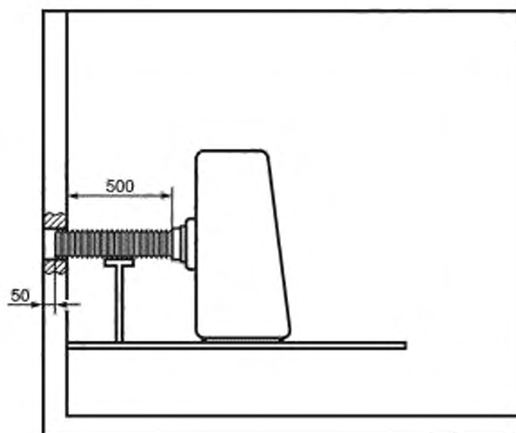
Рисунок A.1 — Типовая установка воздухопроводов
