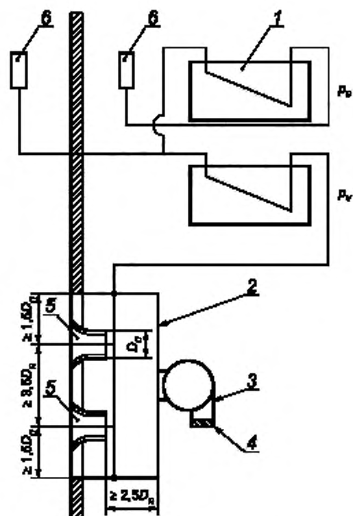
Рисунок С.3 — Устройство выравнивания давления
