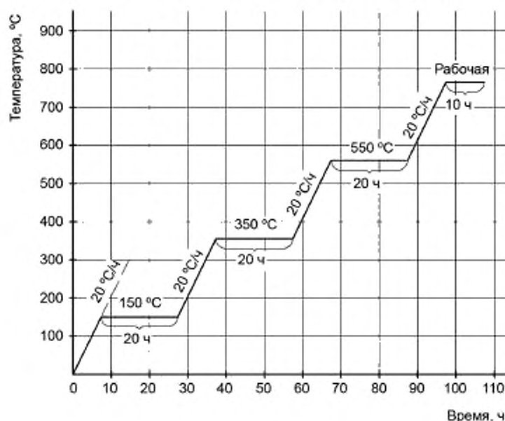
Рисунок 13 — График сушки
