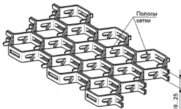
Рисунок 1 — Панцирная гексагональная сетка
