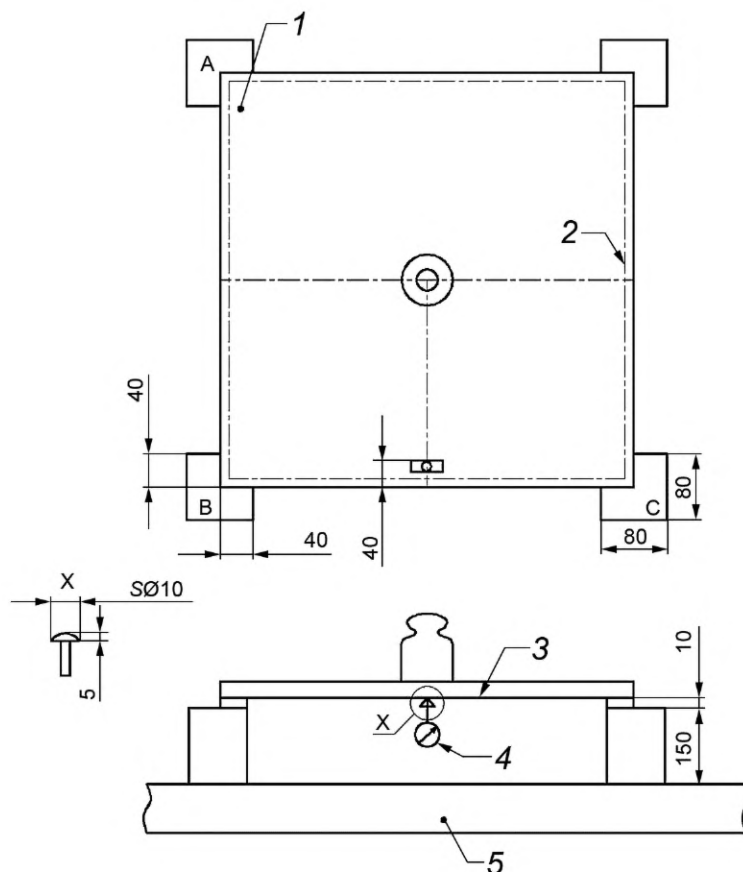
1 — панель; 2 — отделка периметра; 3 — верхняя сторона панели; 4 — индикатор часового типа; 5 — измерительный стол
