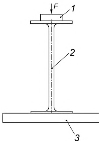
1 — индентор 50×50 мм; 2 — стойка; 3 — станина
