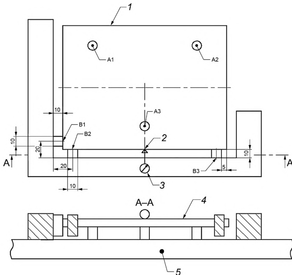
1 — панель; 2 — фронтальная кромка измерительного стержня индикатора диаметром 5 мм; 3 — индикатор часового типа; 4 — нижняя сторона панели; 5 — измерительный стол; A1...A3 — опоры, B1...B3 — поперечные упоры
