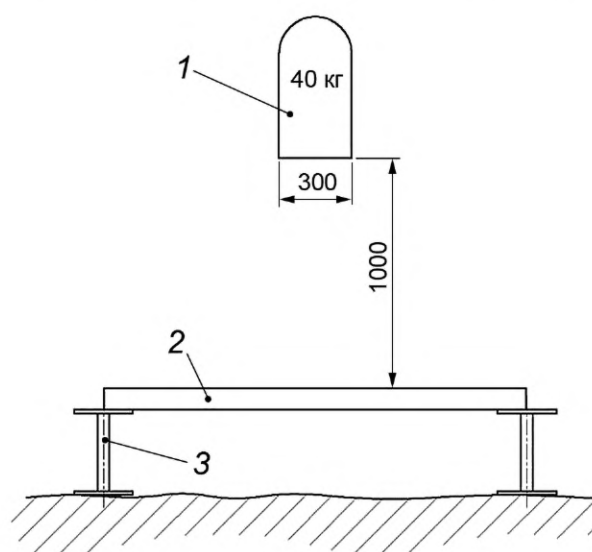
1 — мешок с песком; 2 — панель; 3 — стойка
