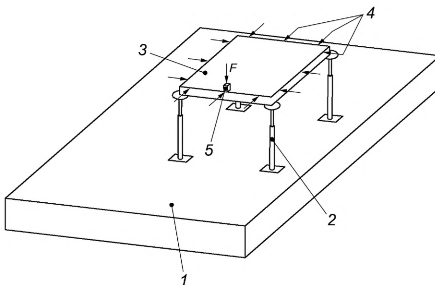
1 — станина; 2 — стойка; 3 — панель; 4 — жесткая рама; 5 — индентор 25×25 мм; F — нагрузка
