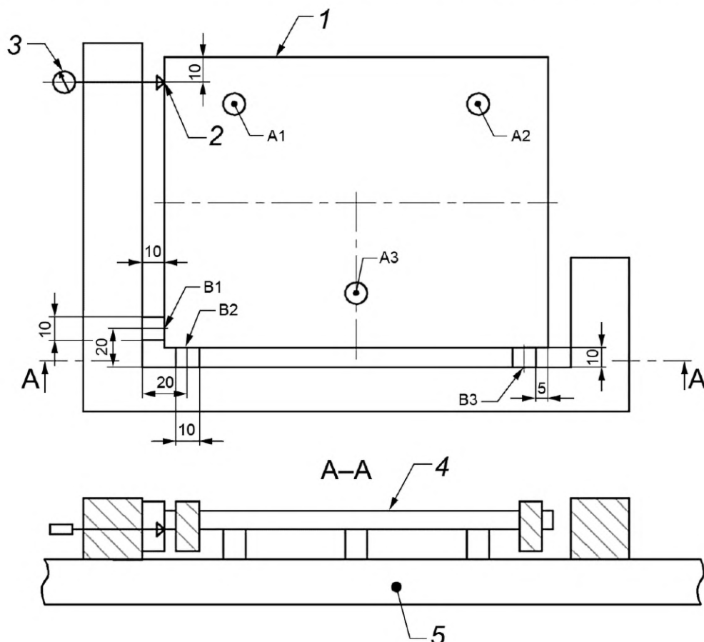
1 — панель; 2 — фронтальная кромка измерительного стержня индикатора диаметром 5 мм; 3 — индикатор часового типа; 4 — нижняя сторона панели; 5 — измерительный стол; A1...A3 — опоры, B1...B3 — поперечные упоры
