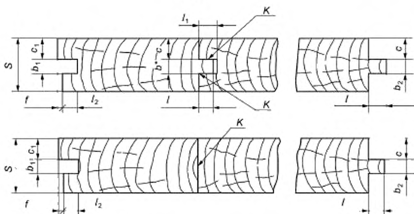
Рисунок 3 — Склейка кромок заготовок щита на гладкую фугу
