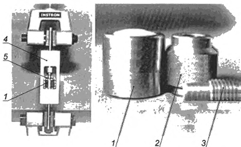
а — многокомпонентная испытательная аппаратура с выровненным образцом в испытательной универсальной машине
