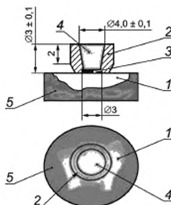
1 — зуб в монтировочном блоке; 2 — форма с заостренным краем; 3 — адгезив; 4 — испытываемый реставрационный материал, помещенный в форму; 5 — монтировочный материал блока (самотвердеющая пластмасса)
