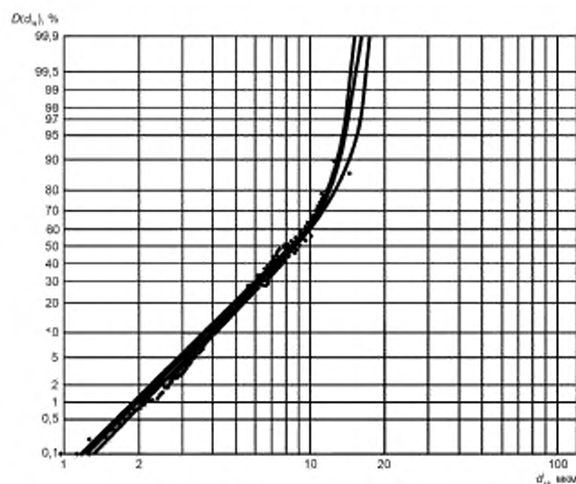
Рисунок Б.2 — Интегральные кривые распределения массы частиц пыли по диаметрам в вероятностно-логарифмической сетке координат
