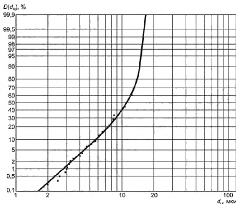
Рисунок А.1 — Результаты определения фракционного состава пыли в выбросе (к примеру расчета массовой концентрации взвешенных частиц PM 2.5 и PM 10 в промышленных выбросах на основе фракционного состава пыли)
