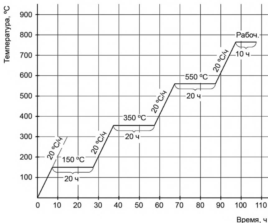
Рисунок 5 — График сушки
