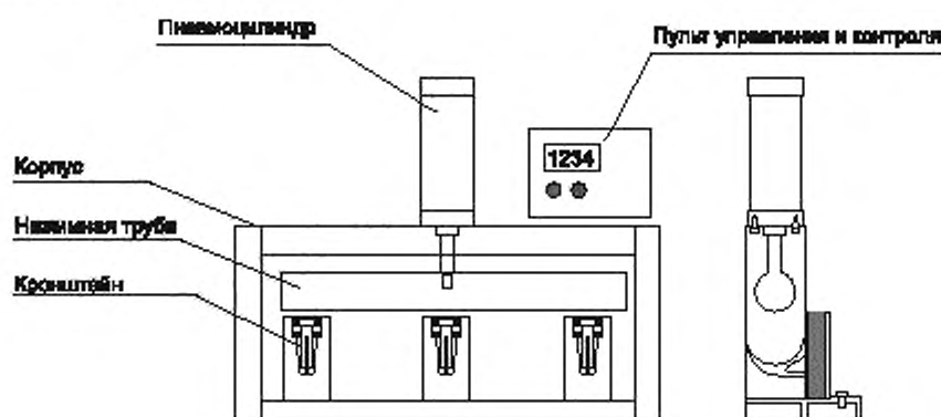
Рисунок 7 — Схема испытательного стенда кронштейнов
