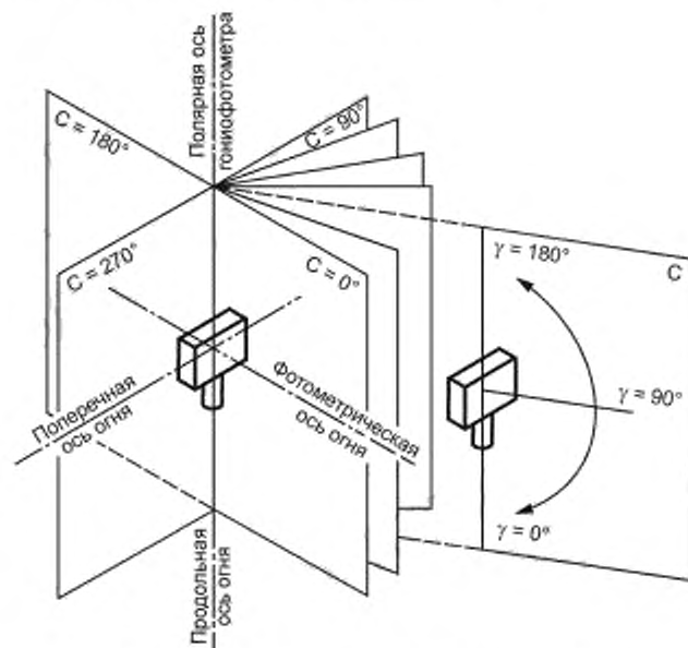
Рисунок В.1 — Система фотометрирования C, \gamma
