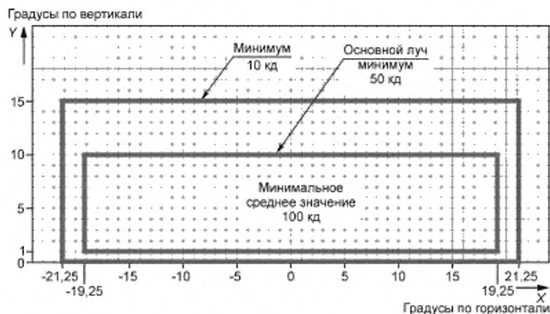
Рисунок Г.13 — Диаграмма изокандел
