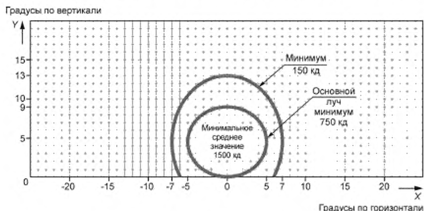
Рисунок Г.19 — Диаграмма изокандел
