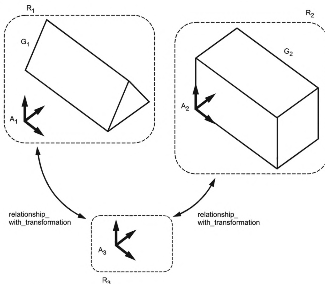
Рисунок 3 — Пример использования объекта representation_relationship_with_transformation
