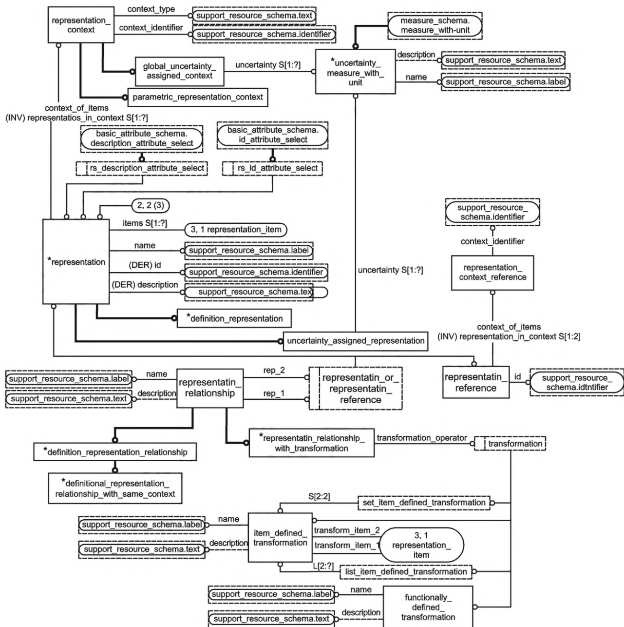
Рисунок D.2 — EXPRESS-G-диаграмма схемы уровня объекта. Диаграмма 2
