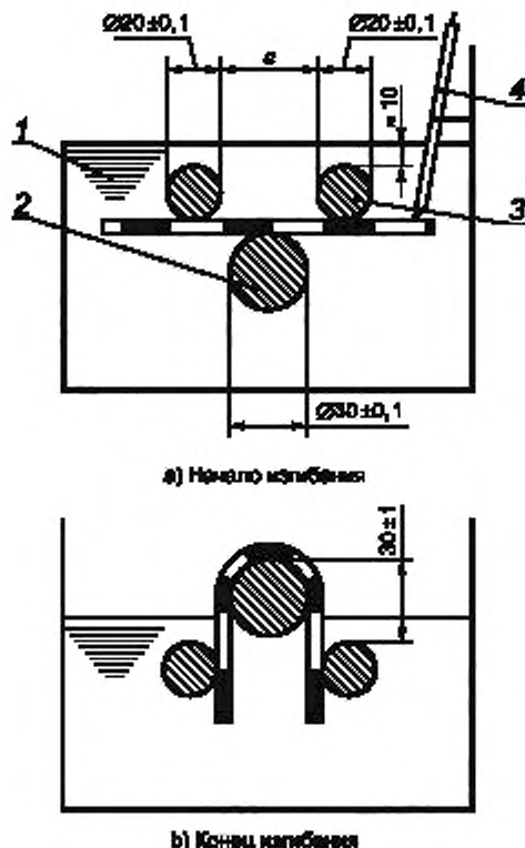
1 — охлаждающая жидкость; 2 — изгибающий стержень; 3 — фиксированный цилиндр; 4 — термодатчик
