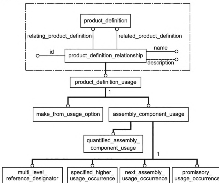
Рисунок 2 — Взаимосвязь объектов структуры изделия по ИСО 10303-41
