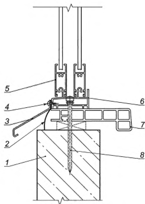
1 — плита железобетонная ограждения балкона; 2 — гидроизоляция; 3 — отлив, 4 — элемент крепления, 5 — сдвижная створка; 6 — рама раздвижной светопрозрачной конструкции; 7 — подоконная доска; 8 — элемент крепления
