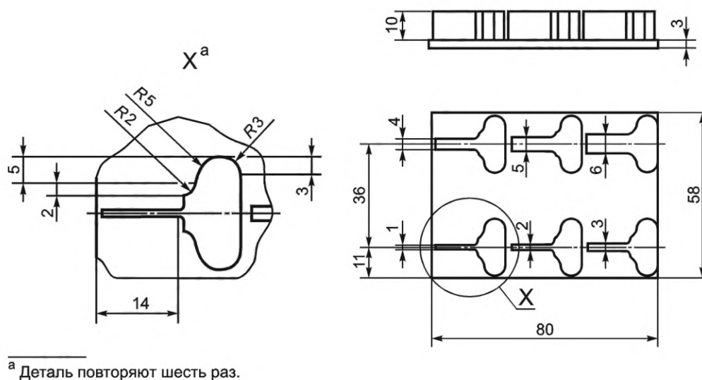
Рисунок 7 — Общий вид крупного элемента с ребрами для определения разрешающей способности
