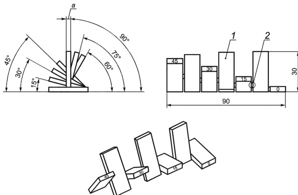
Рисунок 10 — CAD-модели образцов для испытаний структуры поверхности
