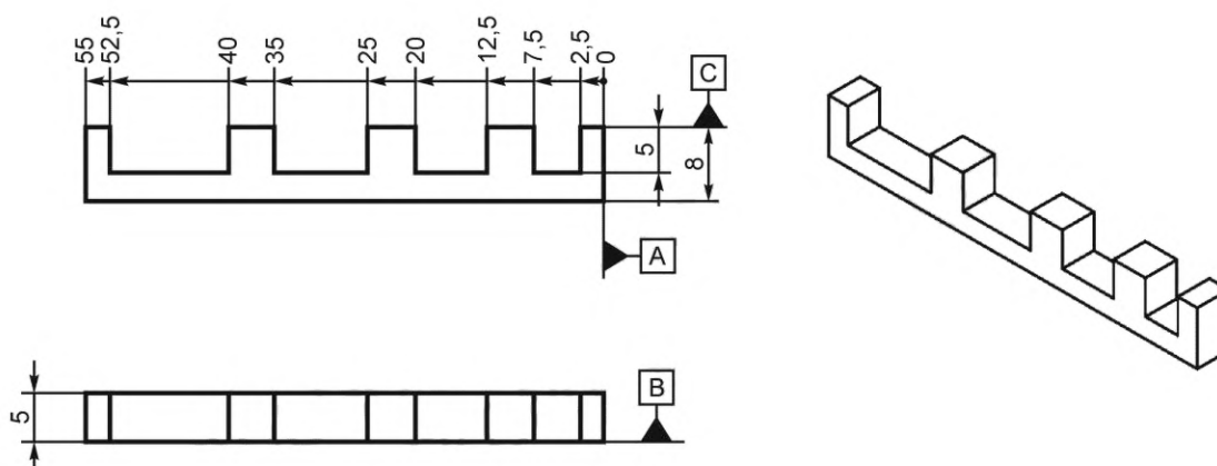
Рисунок 1 — Общий вид линейных образцов для оценки
